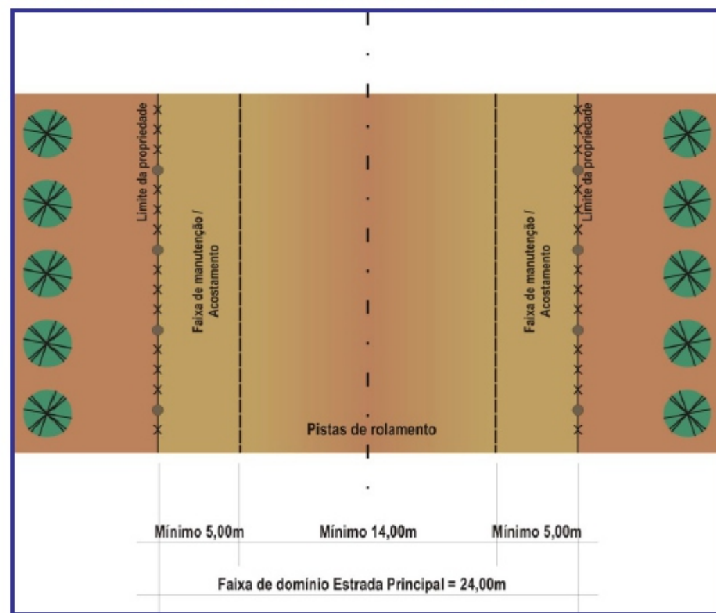
CROQUI ESQUEMÁTICO DA ESTRADA MUNICIPAL RURAL PRINCIPAL
