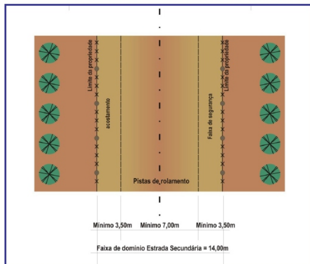
CROQUI ESQUEMÁTICO DA ESTRADA MUNICIPAL RURAL SECUNDÁRIA
