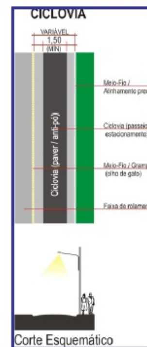
CROQUI E PERFIL ESQUEMÁTICOS DAS CICLOVIAS
